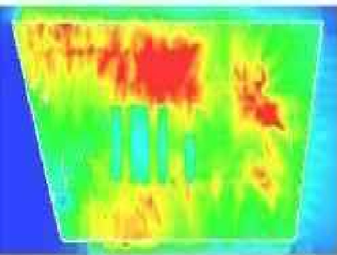
Feux simulés: Température du gaz près du plafond juste avant effondrement
