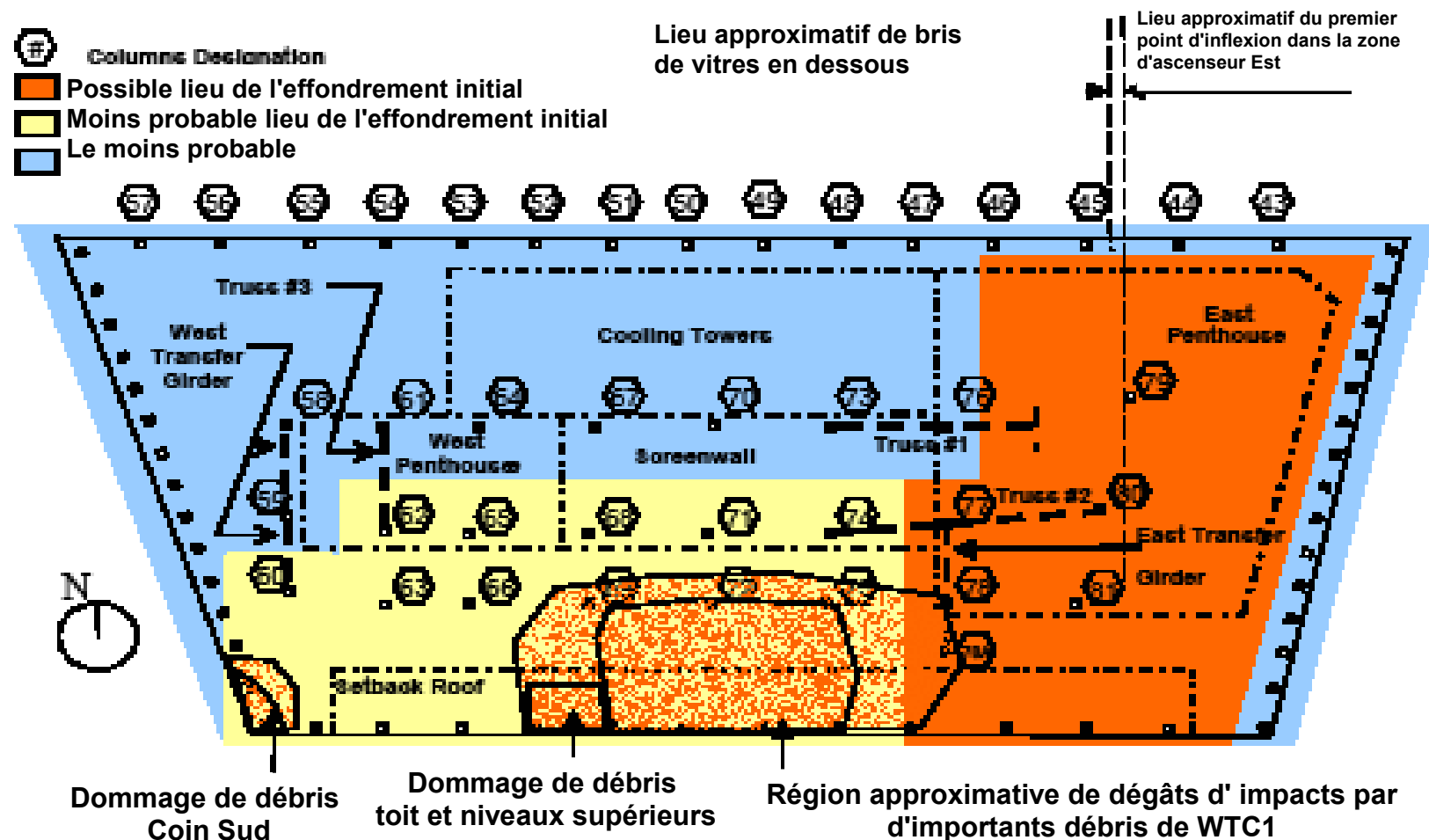
Figure L-29. Vue des zones d'initiation de l'effondrement.
